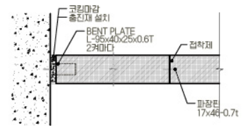
ECO블록 이질재접합 상세도 (평면)
