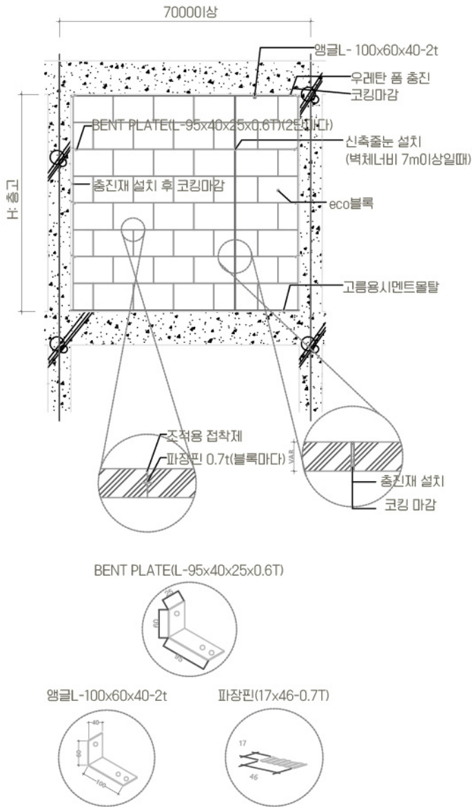
ECO블록 표준 시공 상세도 (입면)
