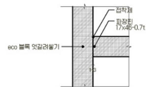
ECO블록 교차부 엇갈려쌓기 상세도-2 (평면)
