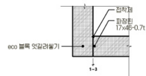
ECO블록 교차부 엇갈려쌓기 상세도-1 (평면)
